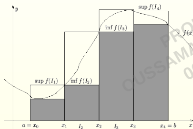
FIG. 1 – Somme de Darboux inférieure (hachurée) et supérieure (hachuré plus blanc) de f(x) pour une subdivision équidistante d'ordre 4 de [a, b] .
